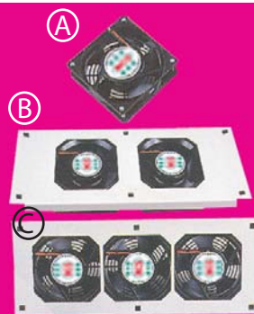
NC-ELF4 : A= 1x4" Fan Part NC-ELF24 : B= 2x4" Fan Part NC-ELF34 : C= 3x4" Fan Part
